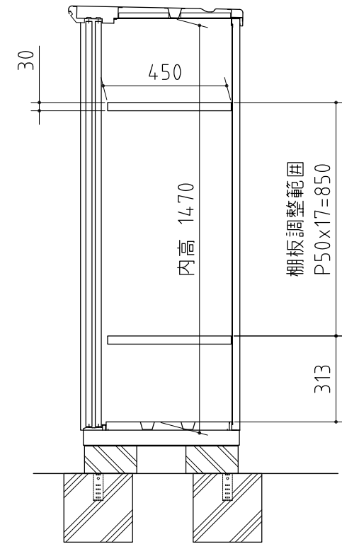
断面図
