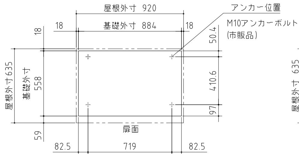
ベタ基礎図
